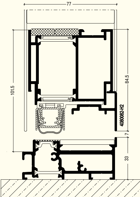
OptiPro Plus DRAAIDEUR
